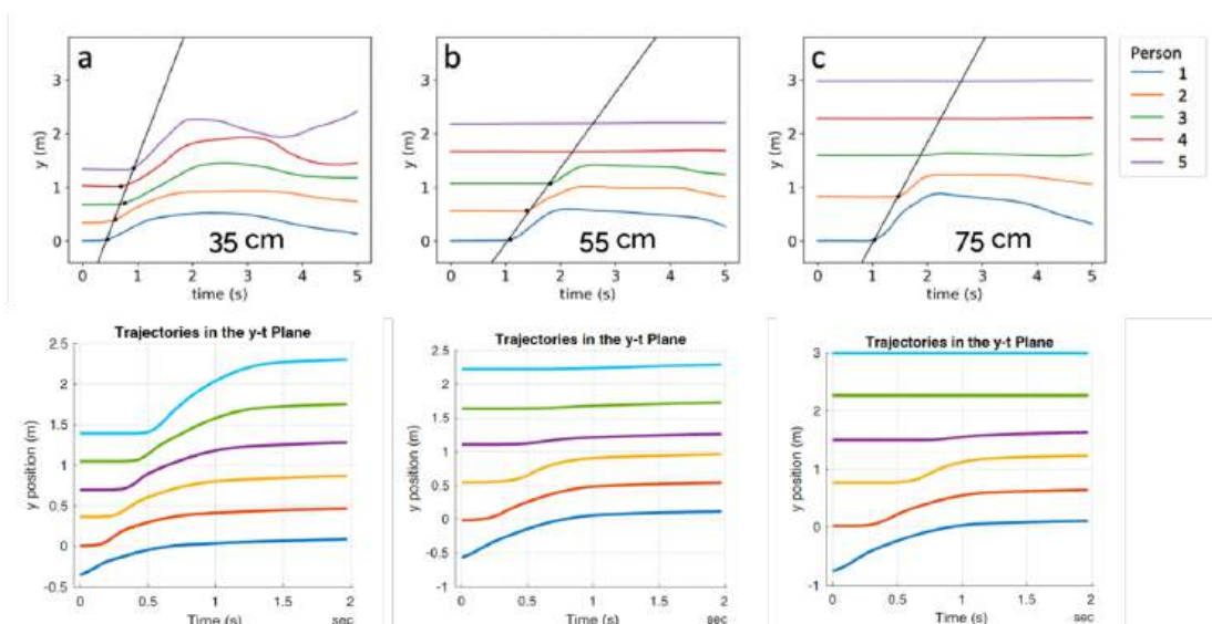
Figuur 14: De resultaten van de modelkalibratie
