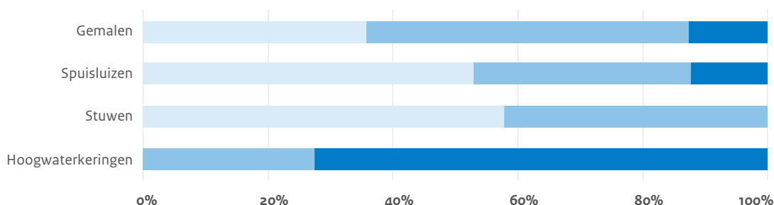
Figuur 9: Levensduur kunstwerken HWS gewogen naar Vervangingswaarde (peildatum: 1 januari 2025).
