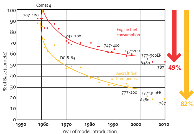
Sinds 1960 is de brandstofefficiëntie van verschillende vliegtuigen sterk verbeterd. Niet alleen het totale brandstofverbruik per vliegtuig is afgenomen, maar ook het brandstofverbruik per stoel.
