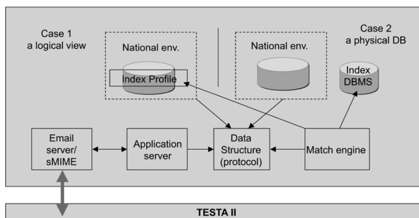
Afbeelding 2: Overzicht van de eigenschappen van de applicatie
